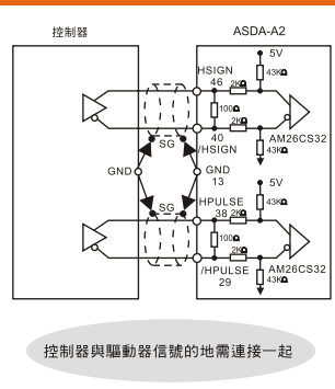
高速脈波命令輸入 (差動輸入)
